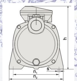
Rozměry čerpadla v mm
